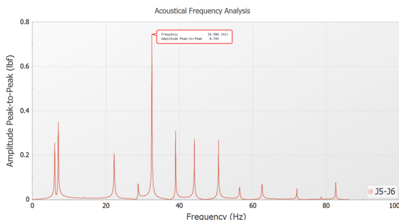
图 7: 声学分析频率图
