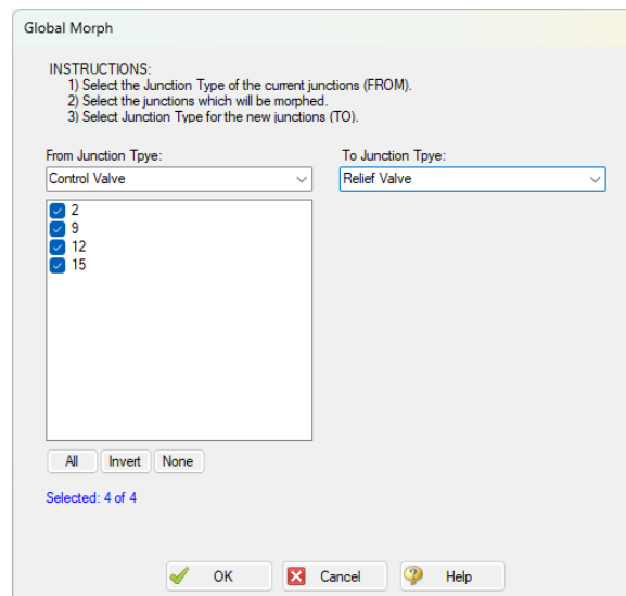
图 11: “全局替换”窗口允许选择同一类型的多个元件转换为另一种元件类型
