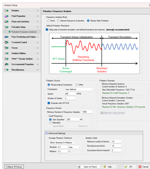
图 6: 分析设置窗口的脉动频率分析面板
