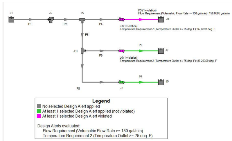
图 4: 工作空间呈现的设计预警图层
