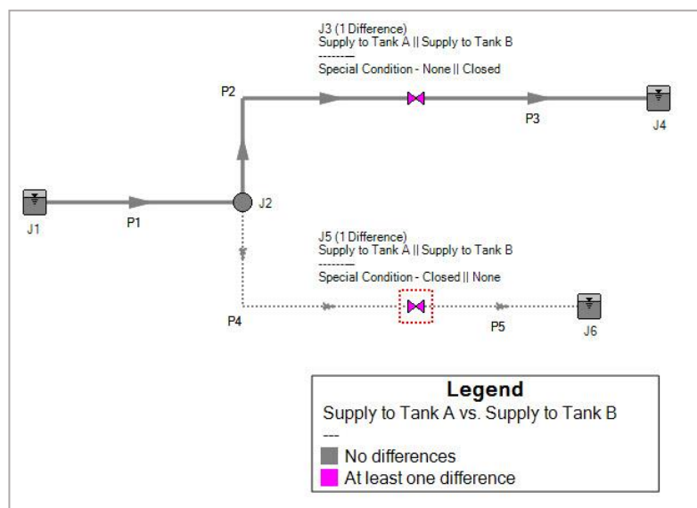
图 5: 工作空间呈现的场景对比图层
