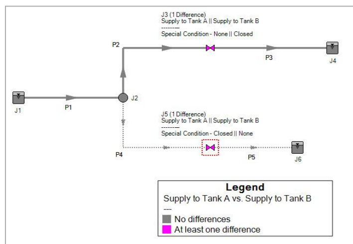
图 4: 工作空间呈现的场景对比图层
