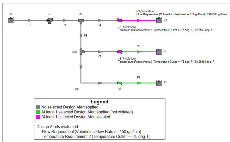
图 7: 工作空间呈现的设计预警图层
