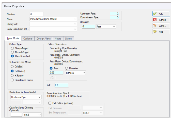
图 6: 孔板属性对话框
