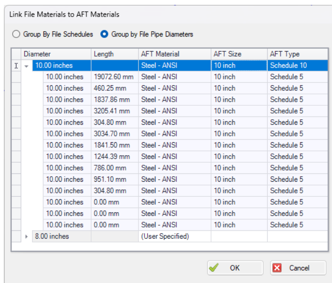
图 9、10 & 11: PCF 导入的新窗口
