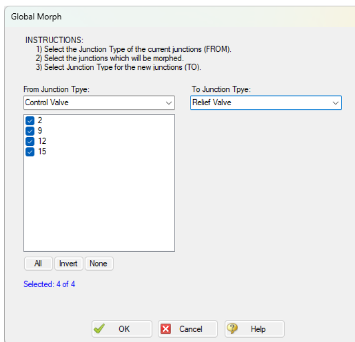
图 12: “全局替换”窗口允许选择同一类型的多个元件转换为另一种元件类型
